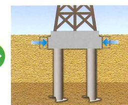
杭の引抜き支持力を期待した場合
