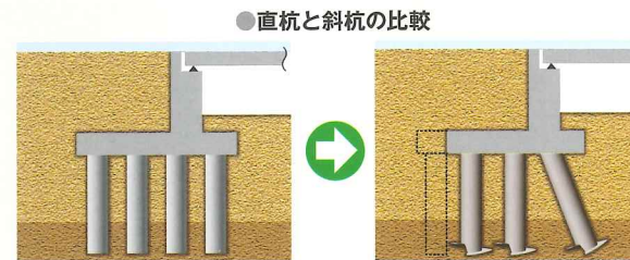
適用可能範囲 傾斜:10°程度以下
